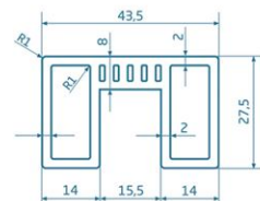
LISTWA OGRODZENIOWA C 1750 X 27,5 X 43,5 MM
