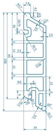
PROFIL ELEWACYJNY 106 X 24 MM
