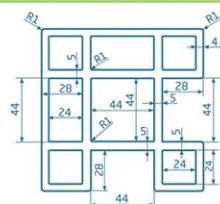
SŁUPEK OGRODZENIOWY NAROŻNY 110 X 110 MM
