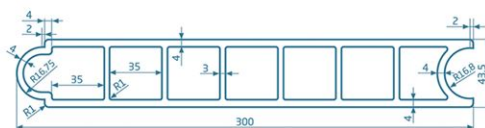
PROFIL OGRODZENIOWY 1950 X 300 X 43,5 MM
