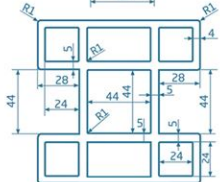
SŁUPEK OGRODZENIOWY 110 X 110 MM
