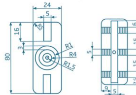
KLIPS + WKRĘT PRESTIGE
